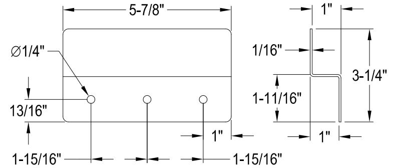
VSPBRKT x 2 pcs (Scale 3:1)
